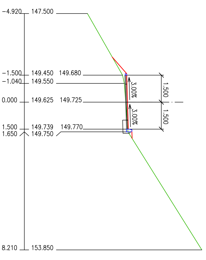
ŘEZ A2 km 0.100000 1:100
