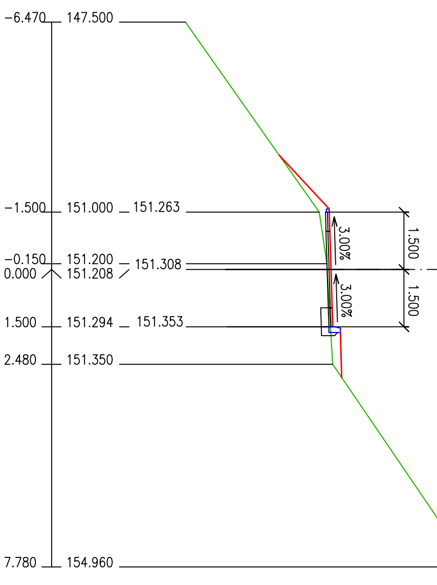
ŘEZ A4 km 0.300000 1:100
