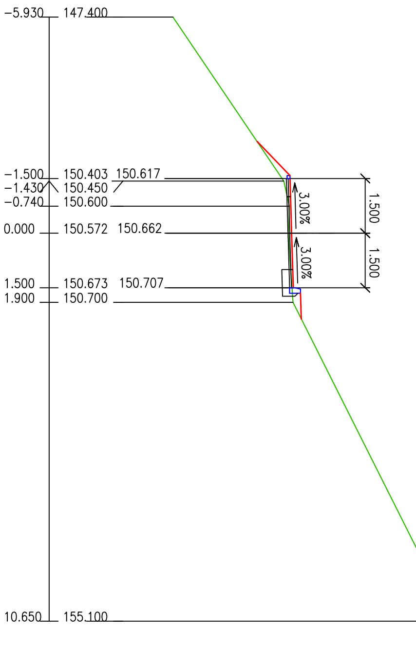
ŘEZ A3 km 0.200000 1:100
