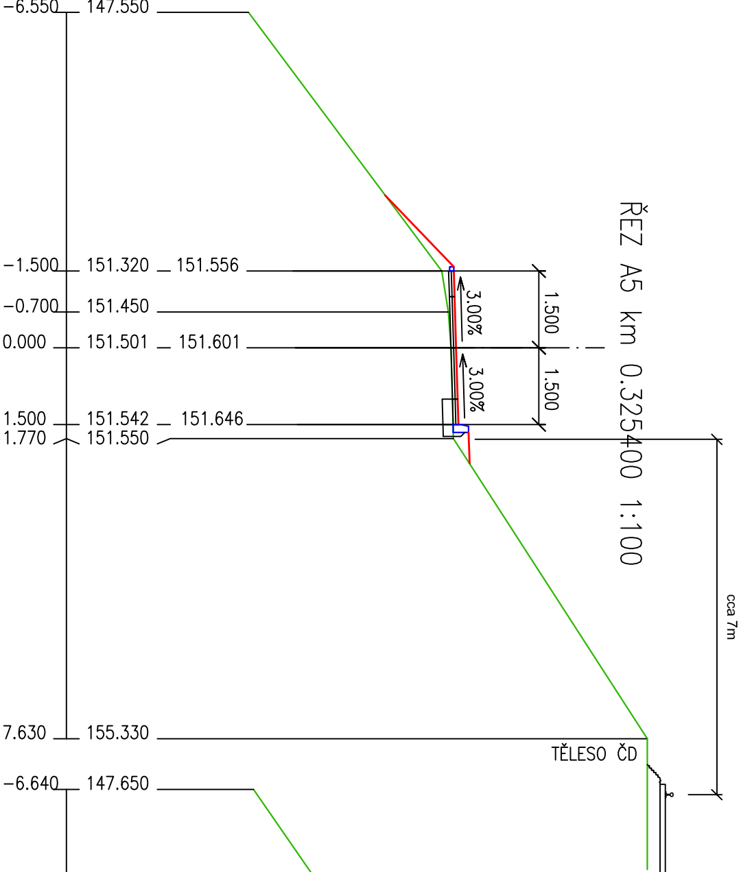
ŘEZ A5 km 0.400000 1:100
